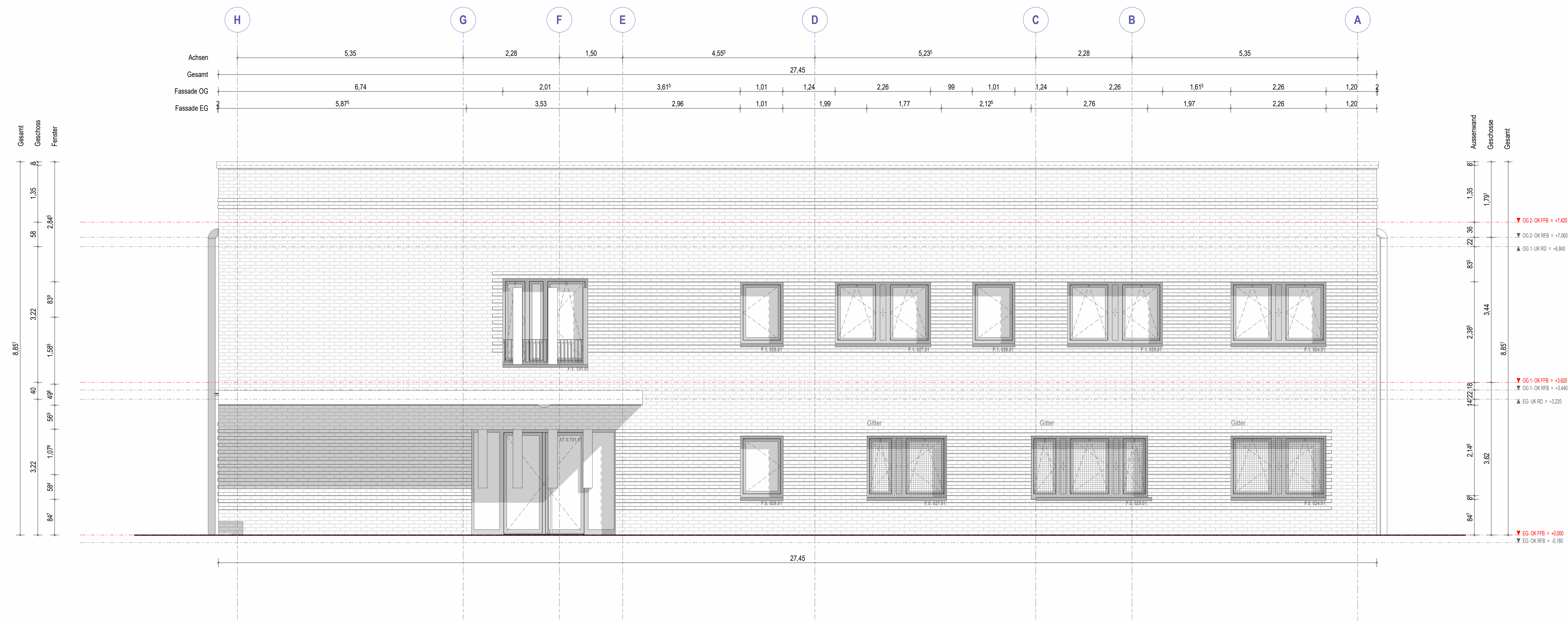
Ansicht Nord
